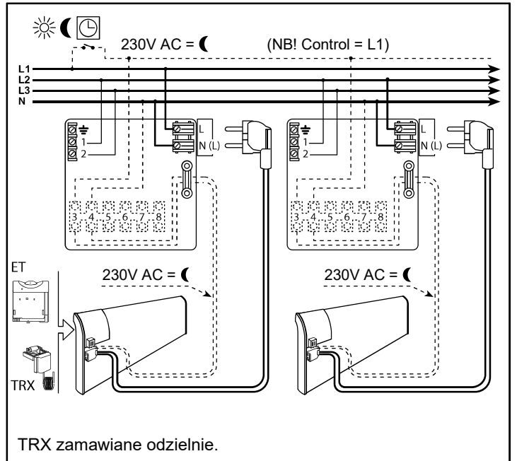
230 woltowy wykres
